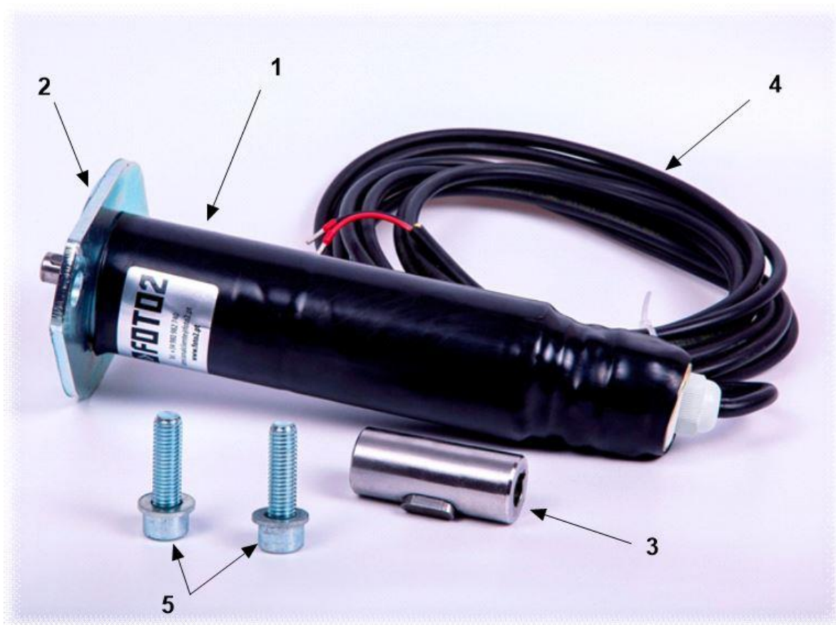
Motor-reductor DC 24V com proteção termo-retrátil
